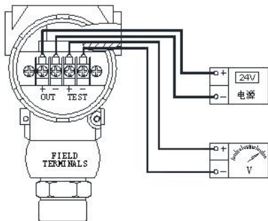
图 5 电压输出
