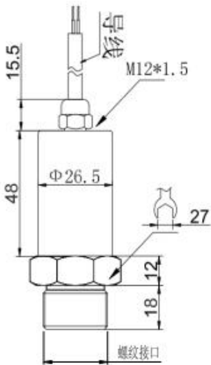
图 2 直接引线型
